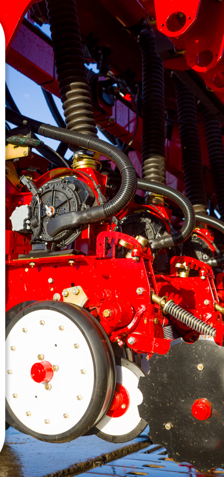
Rueda tapadora de caucho banda trapezoidal con disco escotado
